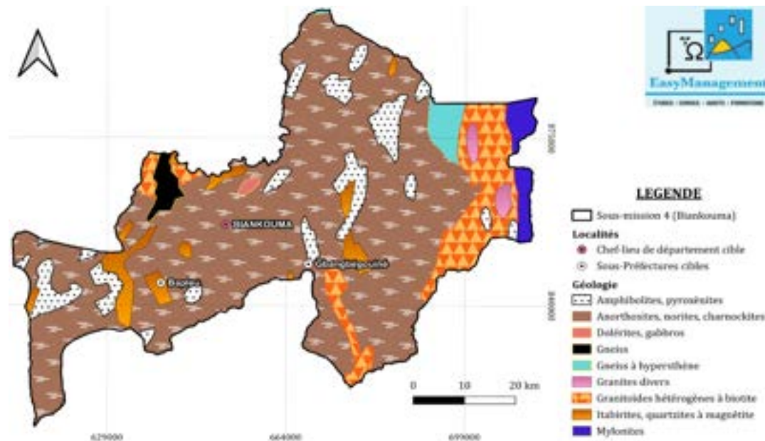
Carte 30: Carte pédologique du Département de Biankouma
