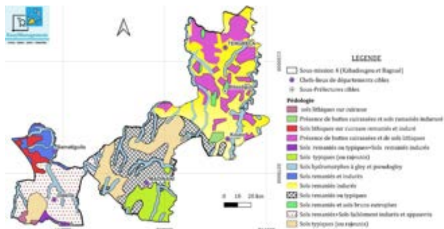
Carte 33 : Carte pédologique de la région du Kabadougou et de la Bagoué
