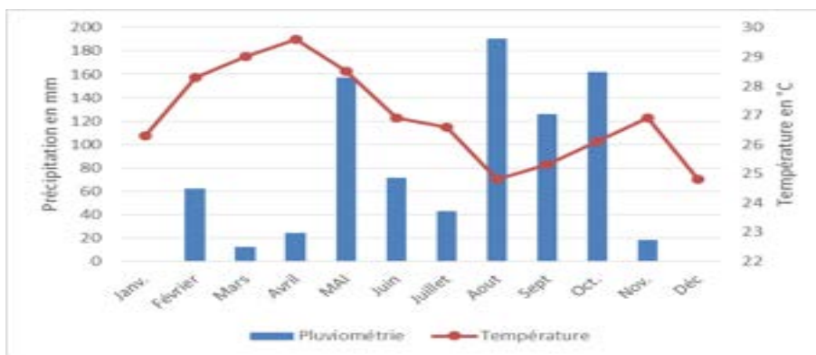
Figure 6: Pluviométrie et température moyennes annuelles
