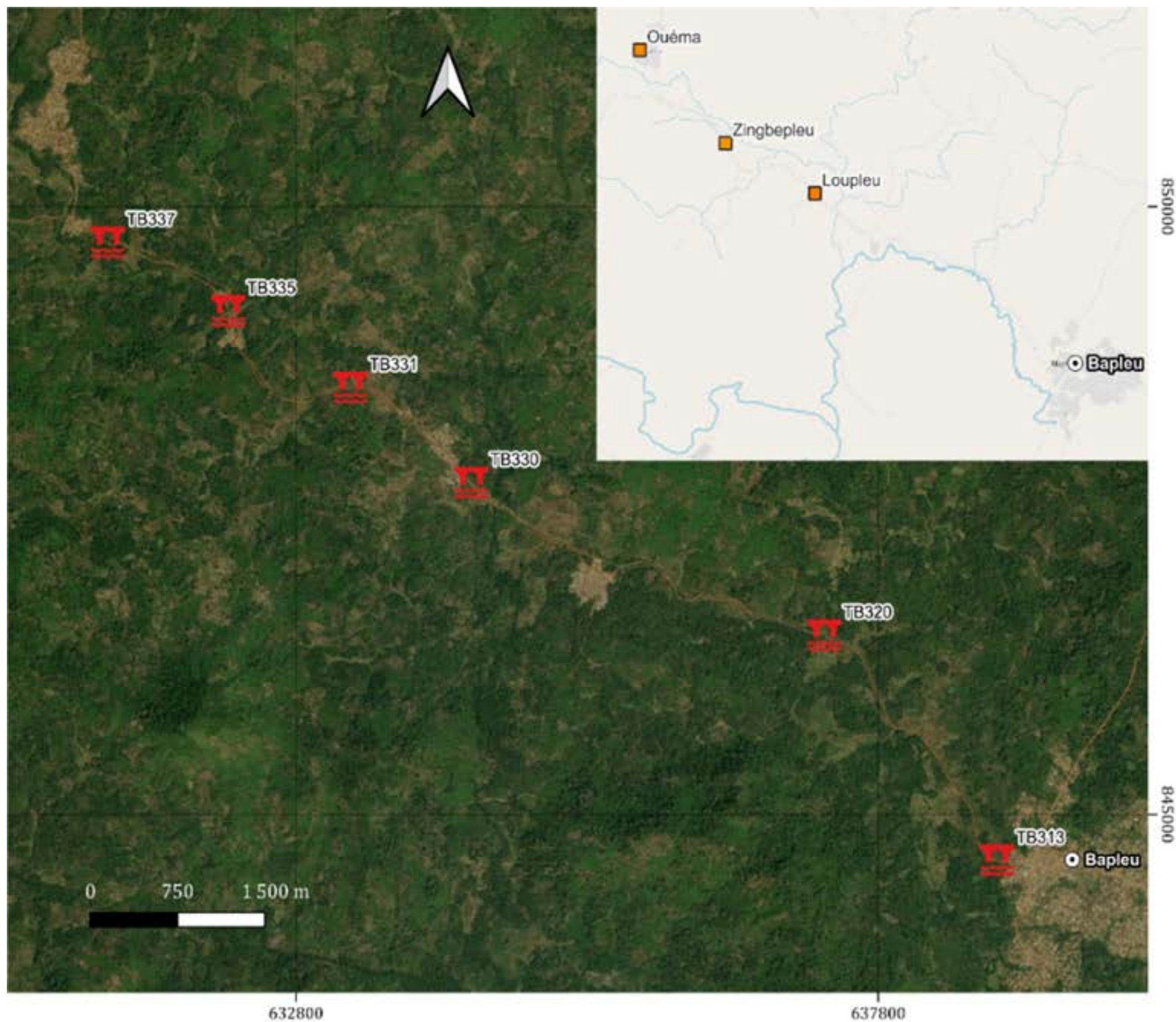
Carte 18 : Localisation des ouvrages hydrauliques à réaliser sur l'itinéraire Blapleu-Ouéma
