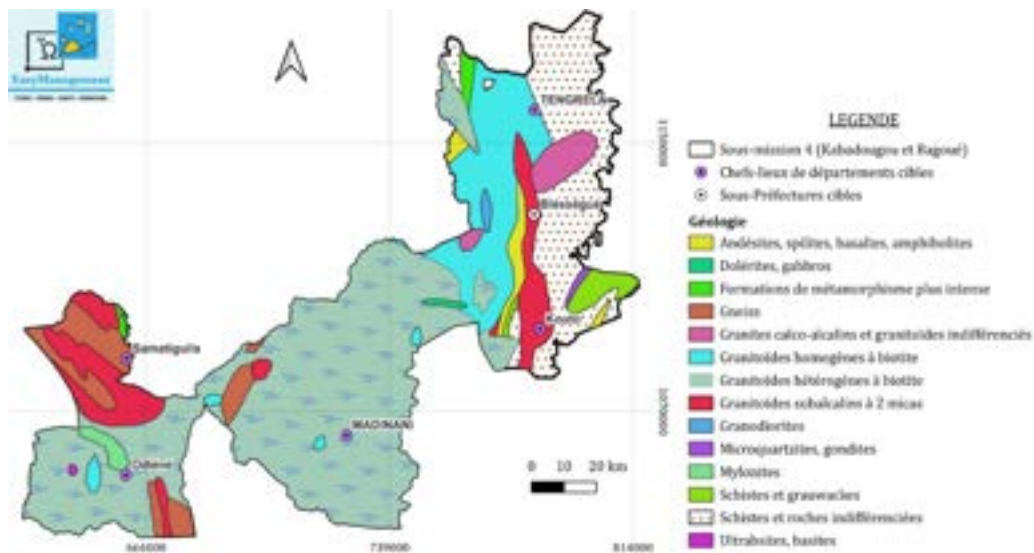
Carte 34 : Carte géologique de la région du kabadougou et de la Bagoué
